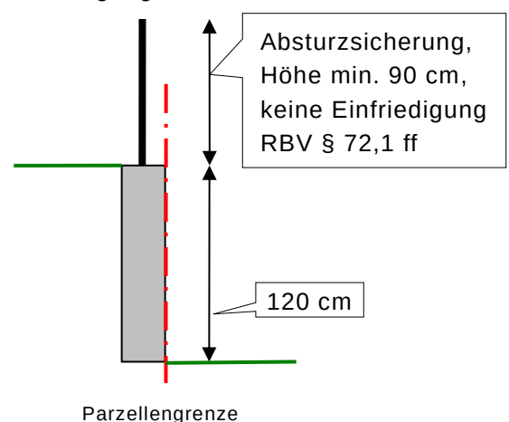
Absturzsicherung bei Stützmauer / Einfriedigung, RBG § 93,2
